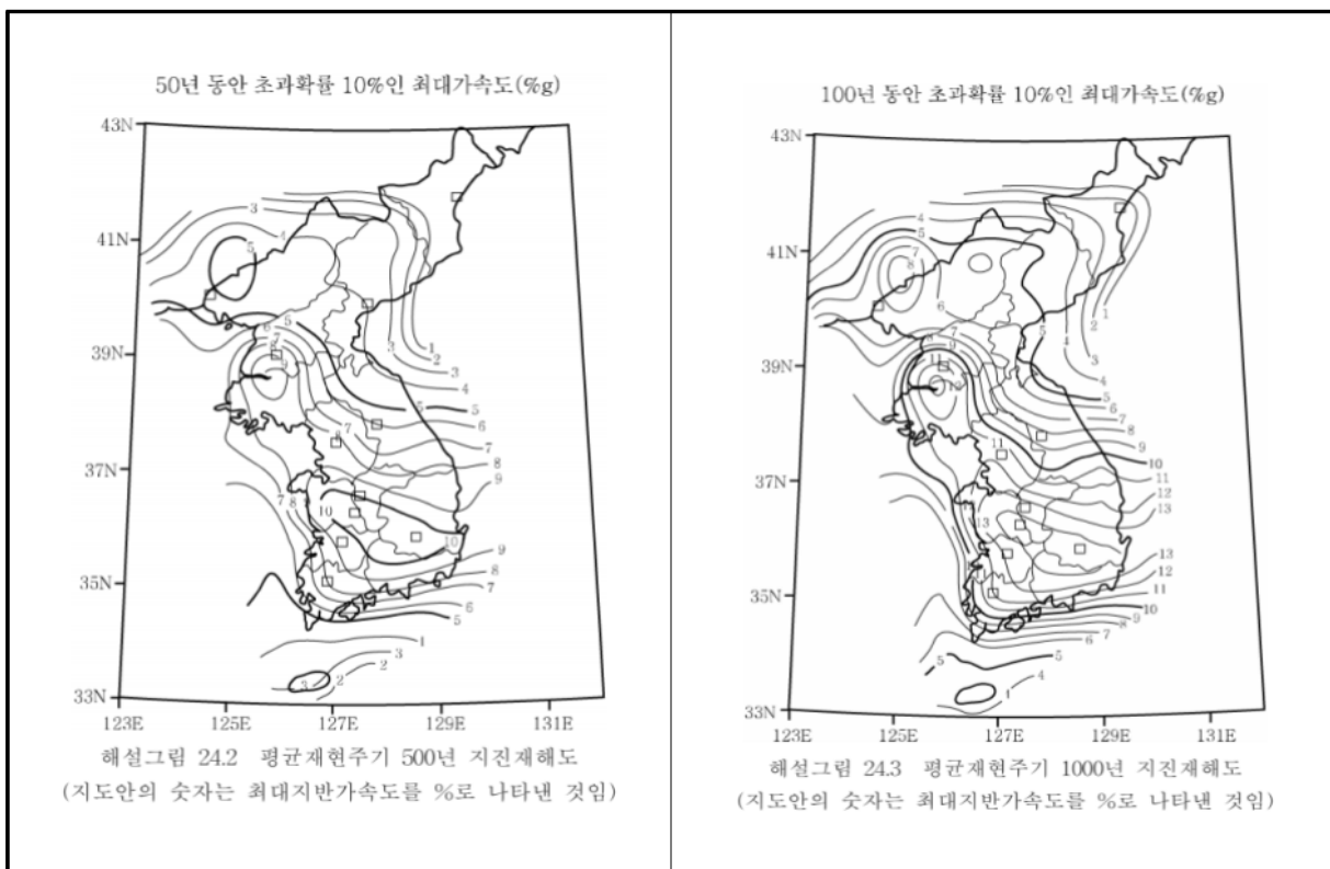
【그림 31.12】 평균재현주기 500년 및 1000년 지진재해도
