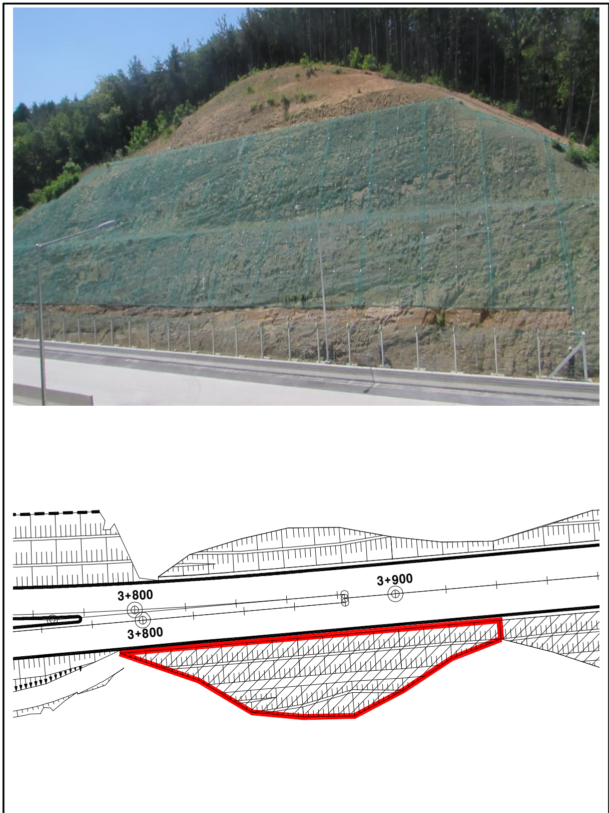
【그림 31.14】 영천절토31 검토대상 비탈면구간
