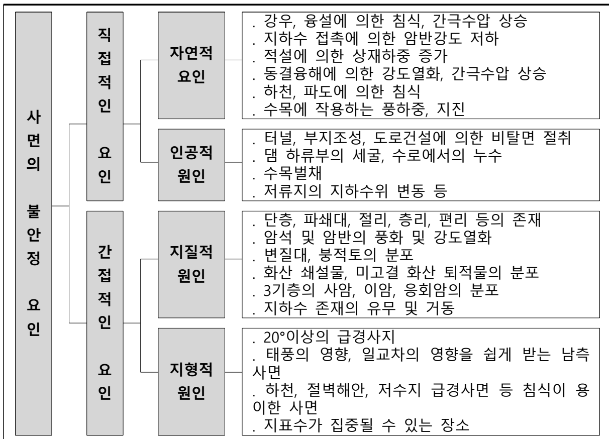
【그림 31.6】 구조안전성능 평가과정
